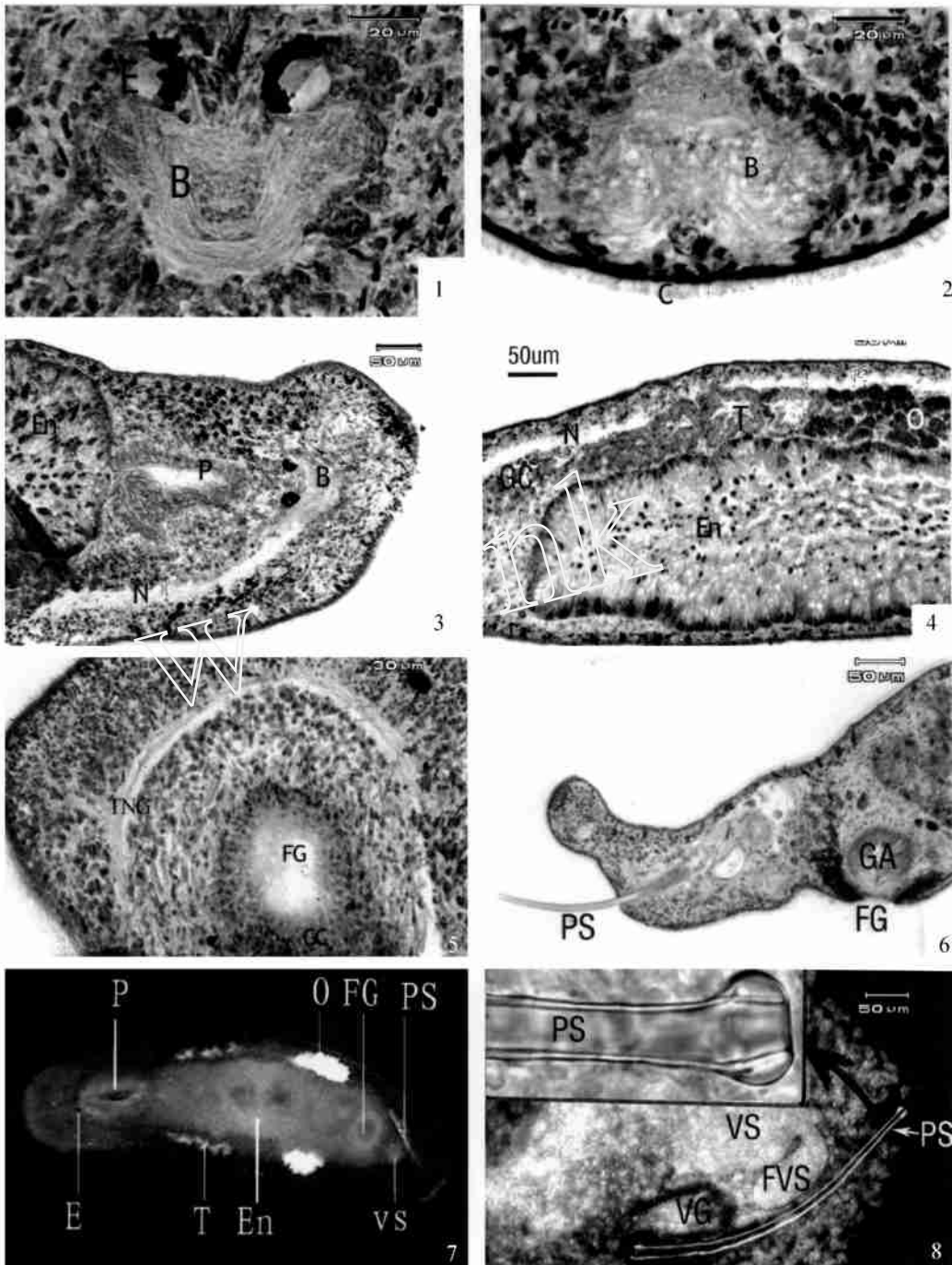
1. 管大口涡虫头部水平切面; 2. 管大口涡虫头部横切; 3. 管大口涡虫身体前部水平切面; 4. 管大口涡虫身体前中部水平切面; 5. 管大口涡虫尾部水平切面; 6. 管大口涡虫尾部纵切; 7. 刚刚麻醉的管大口涡虫; 8. 管大口涡虫雄性生殖器压片。B: 脑; E: 眼; C: 纤毛; N: 神经; P: 咽; En: 消化道; T: 精巢; O: 卵巢; TNG: 尾神经节; FG: 雌孔; CC: 腺细胞; GA: 生殖腔; PS: 阴茎刺; VS: 储精囊; FVS: 假储精囊; VG: 颗粒囊
