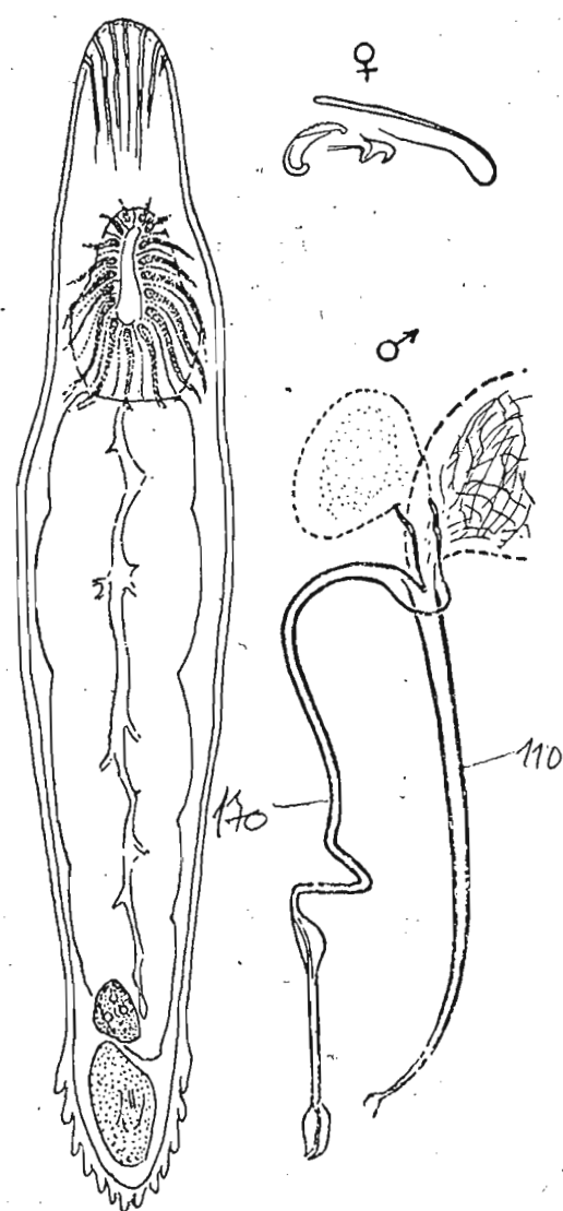
FIG. 3. — Omalostomum ? dubium , n. sp — Individu imparfaitement sexué, \times 150 environ ; ♂, les pièces cuticulaires du pénis à l'état de maturité, \times 500 ; ♀, celles de la bourse copulatrice
